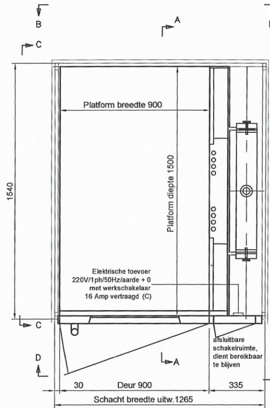
Bovenaanzicht B.G.
