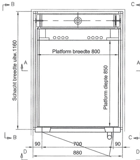
Bovenaanzicht B.G.
